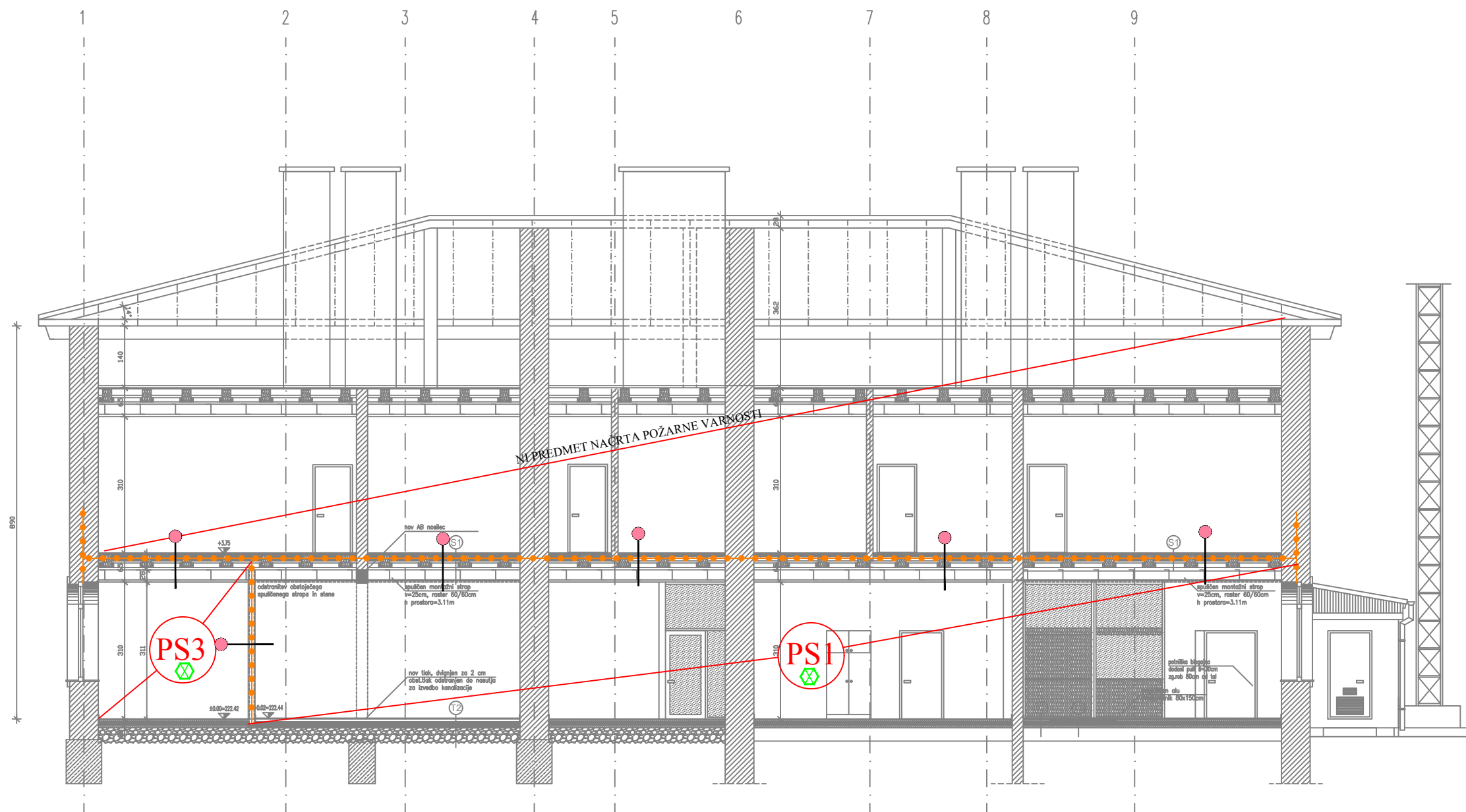
VZDOLŽNI PREREZ A-A POSTAJNEGA POSLOPJA
